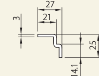
段付寸法
