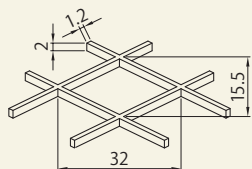
編目寸法
