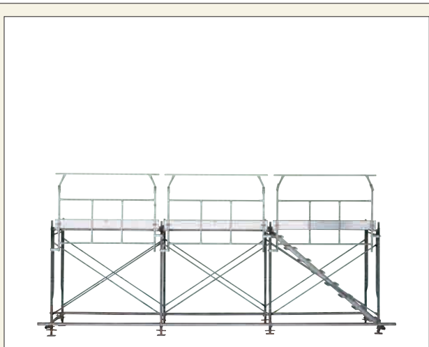
階段枠の取り付け
