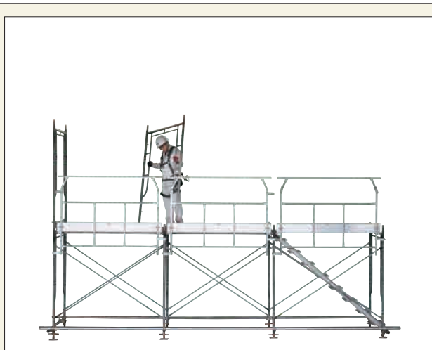
2段目の枠組の配置
