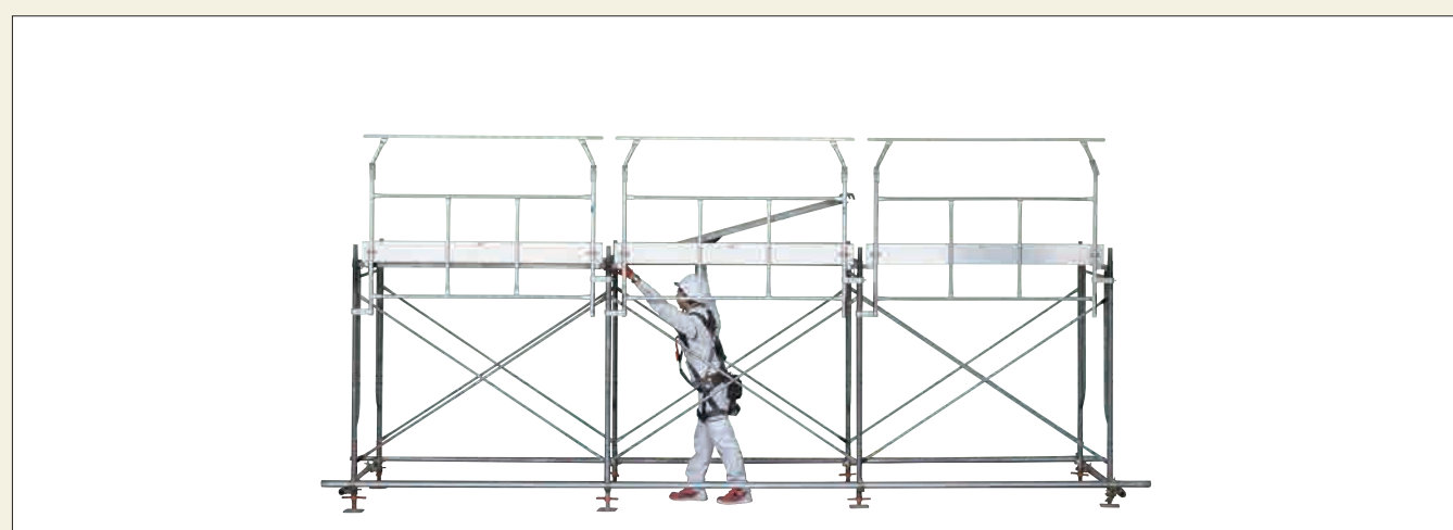
鋼製布板の取り付け
