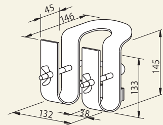
隅梁受 A1453
