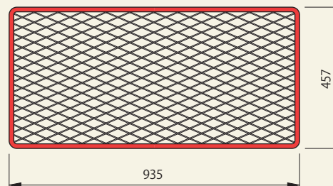
すき間埋め養生板 L型 457・935
