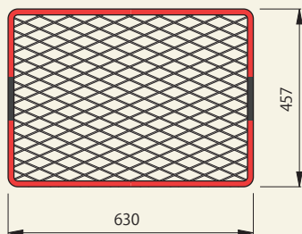
すき間埋め養生板 M型 457・630
