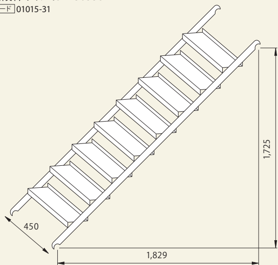
階段枠 アルミSTA3055S
