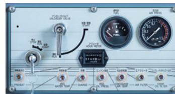
操作パネル
