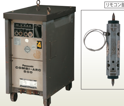
交流アーク溶接機 500Aリモコン付 [コード]03063-52
