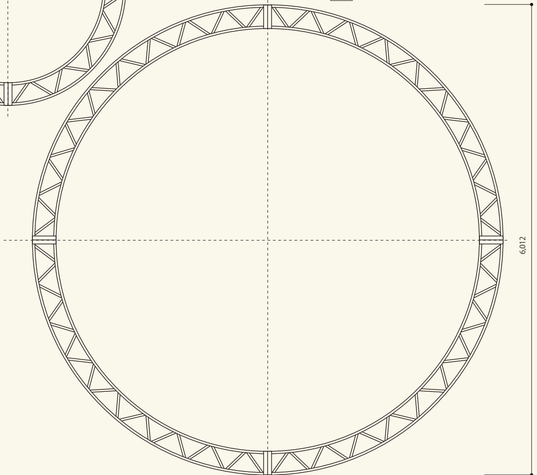
ステージシステム円トラス 直径6m 4分割 サイズ:W4,243×D300×H300 コード 15053-26
