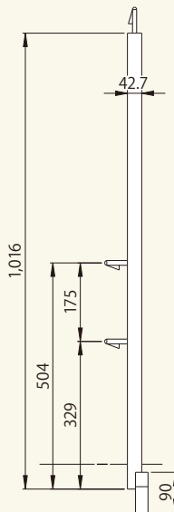
手摺柱N25冠型アームレス タワー枠用 コード|01013-72
