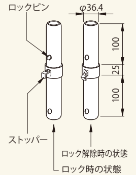
連結ピンアームレス コード|01007-61
