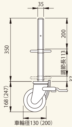
車輪ジャッキ A728 (車輪径200) コード|01011-17
