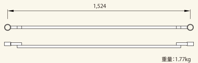
手摺RT4NK タワー枠用 コード|01014-68
