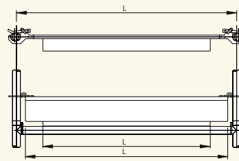
つま先板 L型行止りスチール製 SBH12E
