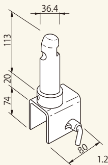
建枠減幅金具 BU-205 [コード] 01007-65
