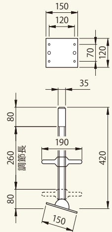
ピボット・ジャッキ [コード] 01011-10
