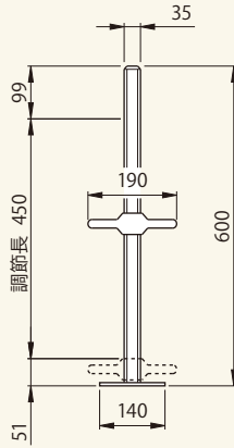
長ベース・ジャッキ [コード] 01011-04
